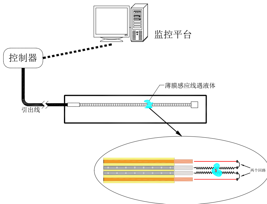
图 1 原理示意图
