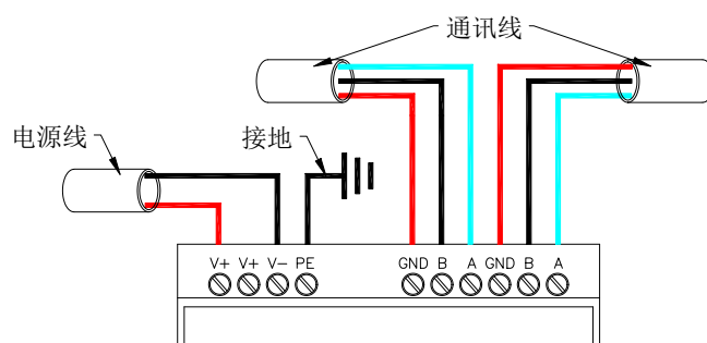
图 5 电源线与通信线连接示意图
