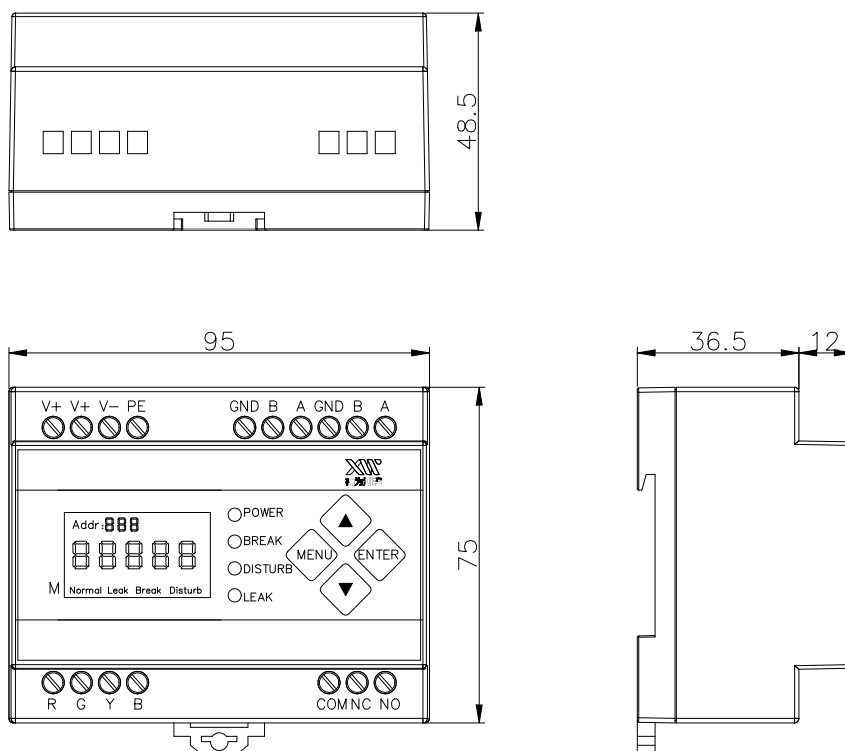
图 1 尺寸图
