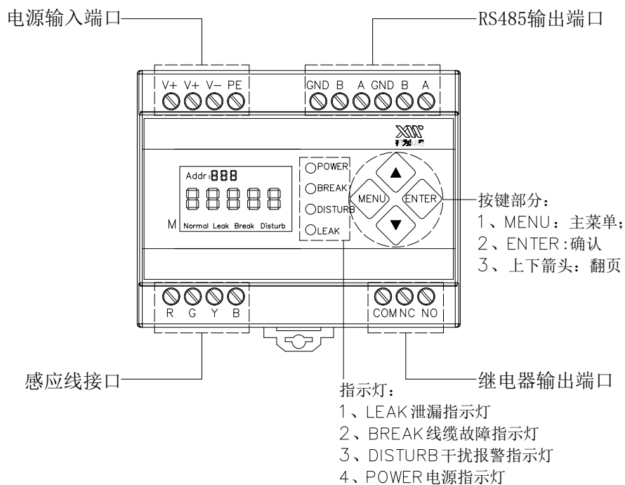
图 2 按键、指示灯与端口说明示意图
