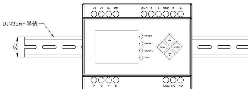
图 4 安装示意图
