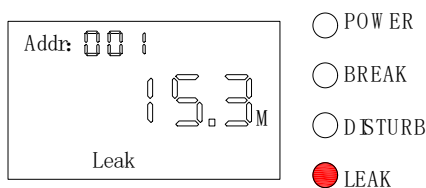
图 10 泄漏状态界面
