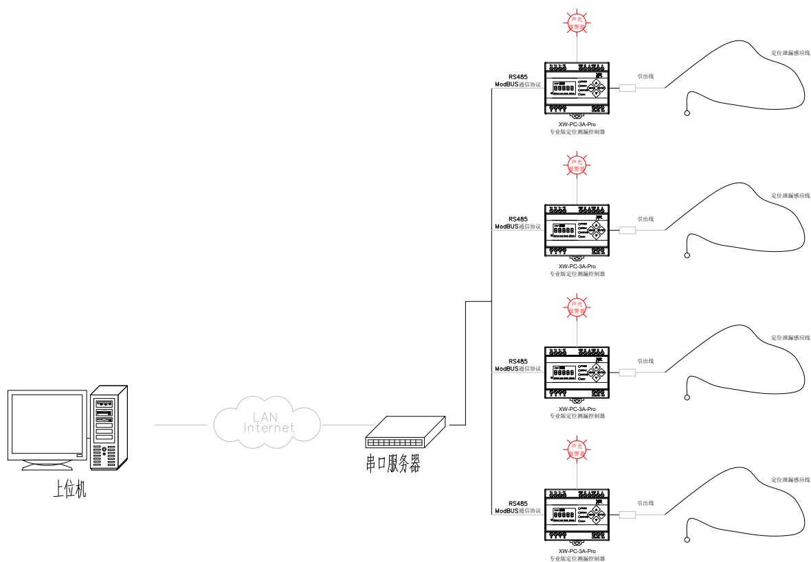
图 3 系统拓扑图
