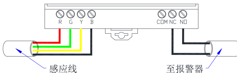
图 6 感应线与继电器连接示意图
