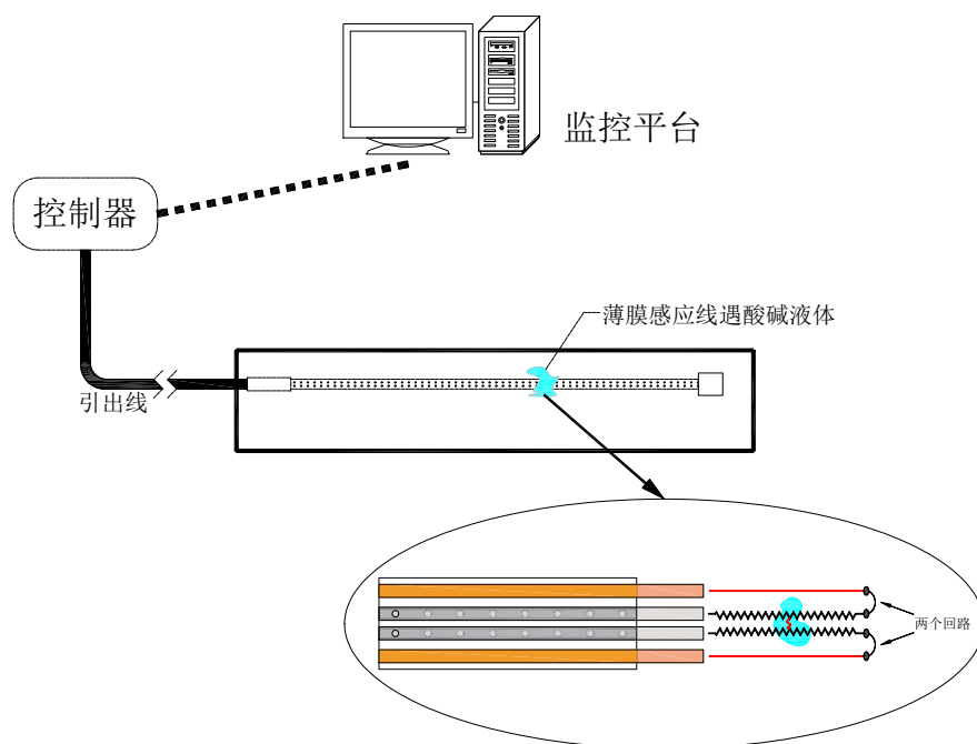
图 1 原理示意图
